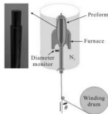
图 3 棒管法拉丝原理图
