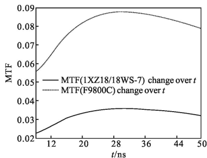
(d) MTF 与选通时间之间的关系 ( f=15 lp/mm)
