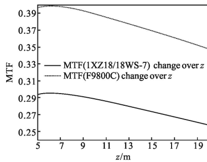
(c) MTF 与探测距离间的关系 ( f=15 lp/mm)
