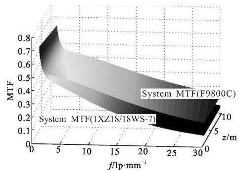
(a) MTF 与空间频率、探测距离之间的关系
