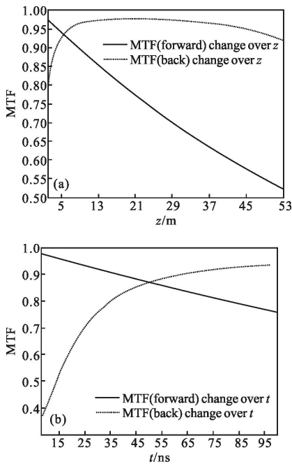
图 5 MTF_{forward} 与 MTF_{back} 随探测距离与时间变化的关系
