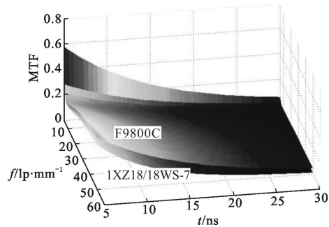
(b) MTF 与空间频率、选通时间之间的关系
