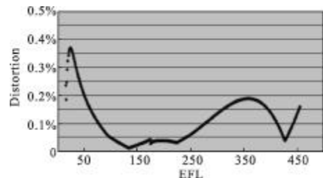
图 9 全变焦范围内畸变变化曲线
