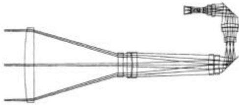
图 3 20×中波红外变焦镜头长焦 400 mm 位置的折叠结构 Fig.3 Folded configuration in f=400 mm of MWIR zoom lens with 20× ratio
