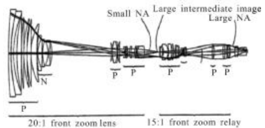
图 14 300×高变焦比系统示意图
