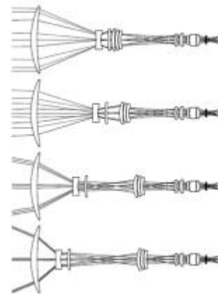
图 7 30×中波红外变焦系统结构图 Fig.7 Schematic of MWIR zoom lens with 30× ratio
