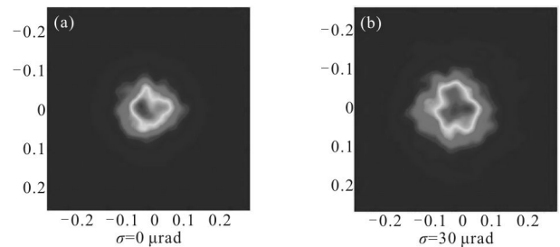
图 3 跟踪抖动与大气湍流综合作用下的积分光斑
