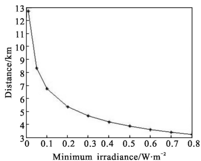
图 3 最小可探测辐照度与作用距离关系
