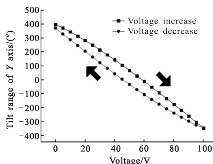
图 8 快速反射镜偏摆范围测试结果
