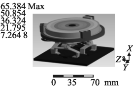
(d) 四阶模态-扭转 (d) 4th mode-torsion
