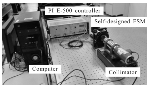
图 7 快速反射镜偏摆范围测试实验设备
