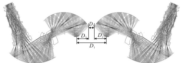
图 9 部分双目重叠双目系统结构
