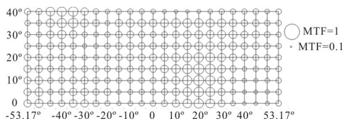
图 6 50\text{lp/mm} 处子午、弧矢平均 MTF
