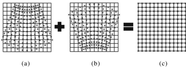
图 3 双椭球反射面的畸变补偿。(a) 椭球 1 引入的畸变; (b) 椭球 2 引入的畸变;(c) 双椭球畸变补偿后的结果
