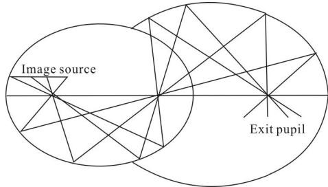
图 2 双椭球反射面成像原理 Fig.2 Double ellipsoidal mirrors imaging principle
