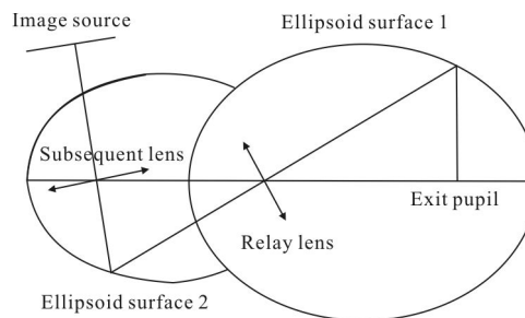
图 1 双椭球结构系统示意图
