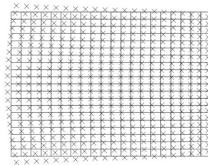
图 7 全视场 106.3^{\circ}(\text{H})\times 80^{\circ}(\text{V}) 范围内的网格畸变
