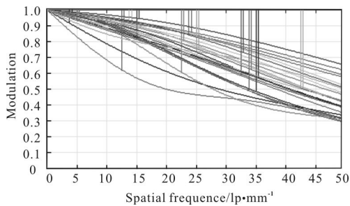
(a) 双自由曲面结构 MTF
