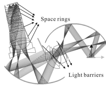
图 8 正向光线传播路径
