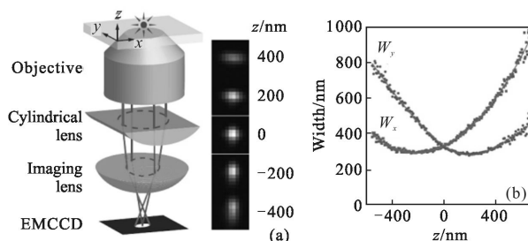
图 4 使用柱面镜精确检测单个荧光团 z 轴位置的 STORM 技术 [7]
