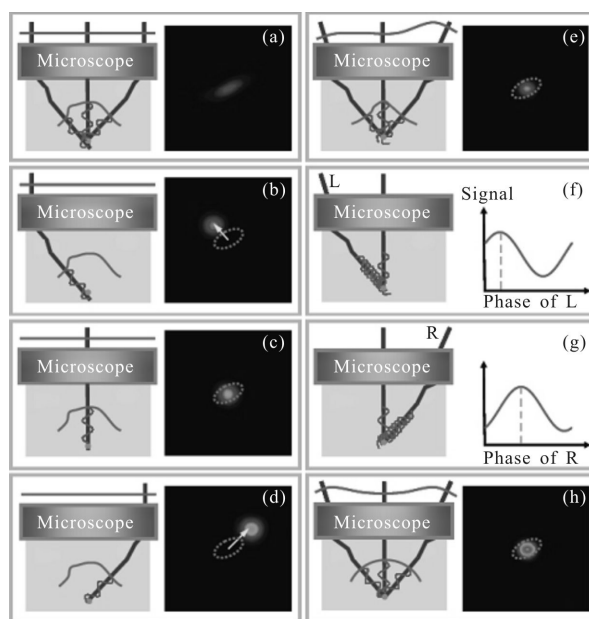
图 7 出瞳面分区域校正轴上点的倾斜波前和共相位波前 [10]
