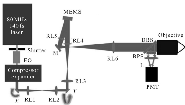
图 9 使用 MEMS 变形镜在多光子点扫描显微镜中校正激发光波前分布 [11]
