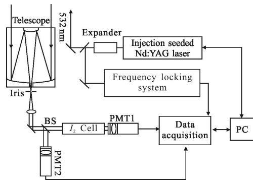
图 3 HSRL 系统结构图
