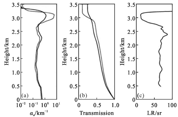
图 4 2015 年 3 月 31 日夜间 HSRL 激光雷达观测结果
