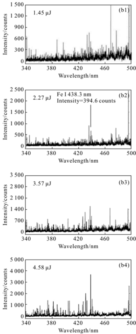
图 6 Al 原子(a)和 Fe 原子(b)的光谱强度图 Fig.6 Spectral intensity of Al atom(a) and Fe atom (b)
