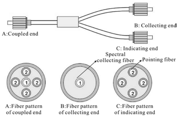
图 2 一分二结构的多芯光纤束
