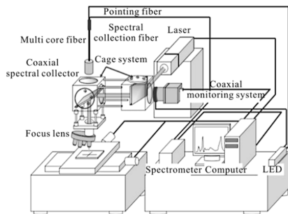
图 1 远场光学激光探针系统结构图
