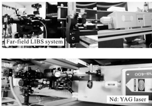
图 5 激光探针装置的侧视图(a)与俯视图(b) Fig.5 Side view (a) and vertical view (b) of LIBS experimental setup
