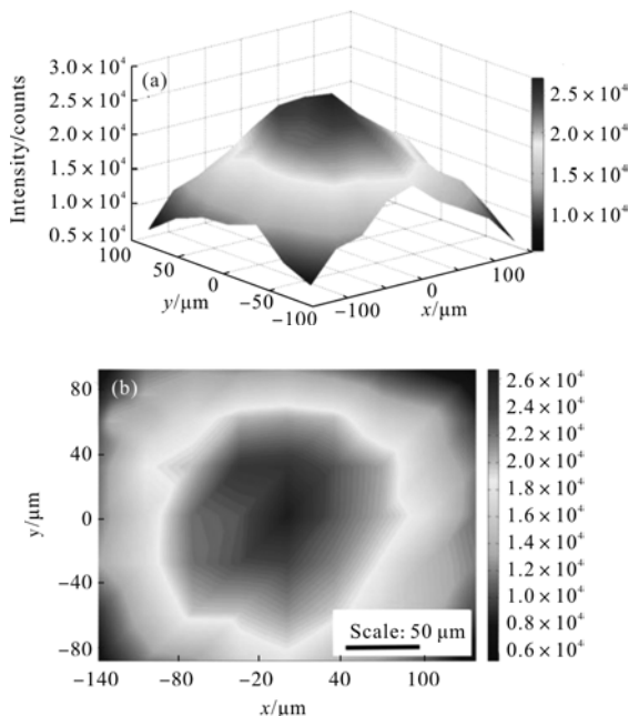
图 10 Al 原子谱线强度的空间三维分布图(a)和 空间二维分布图(b)
