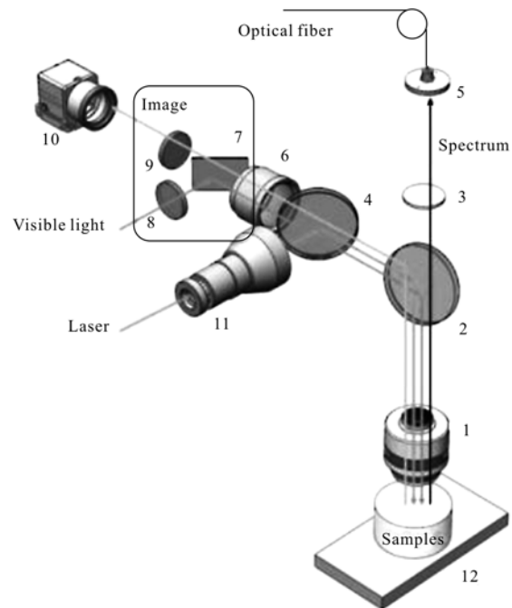
图 3 激光探针光学系统图
