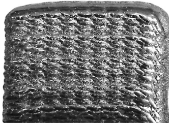
图 4 激光沉积修复试样侧塌边缺陷
