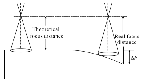
图 6 离焦量对成形高度的影响
