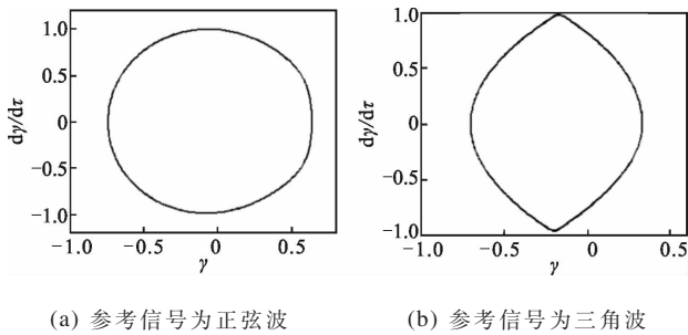
图 4 受控 MOEMS 追踪控制轨迹相图
