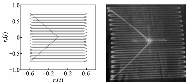
(c) 线性回归指令信号 (d) 线性回归扫描轨迹图 (c) Command signal of linear regression (d) Trajectory diagram of linear regression
