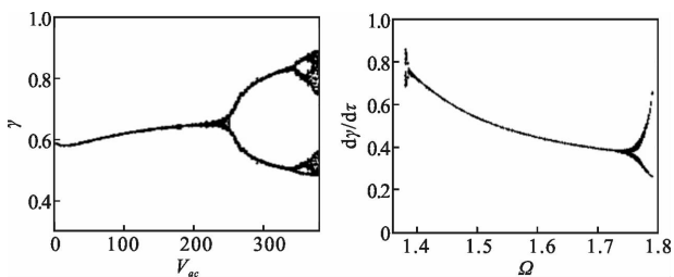
(a) 交流电压幅值
