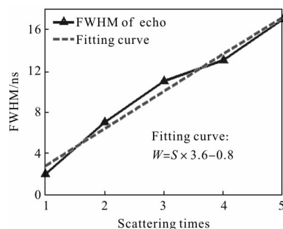
(b) 回波半高宽度与散射次数的关系
