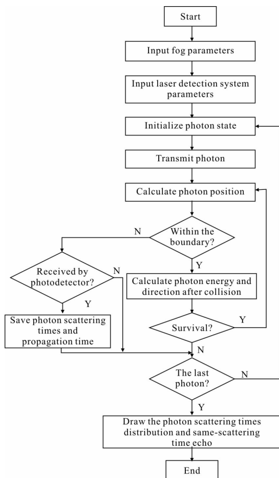
图 1 激光云雾传输模型仿真流程
