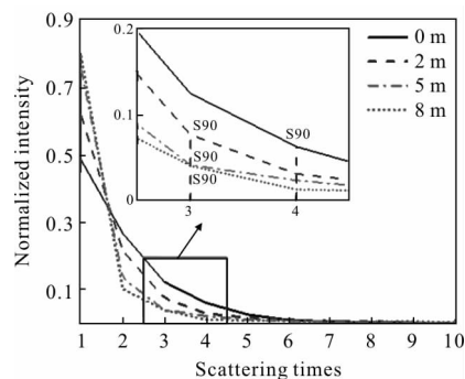
(b) 不同云雾距离
