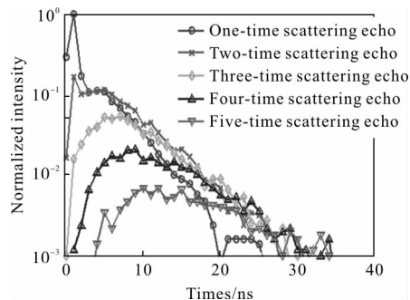
(a) 回波波形
