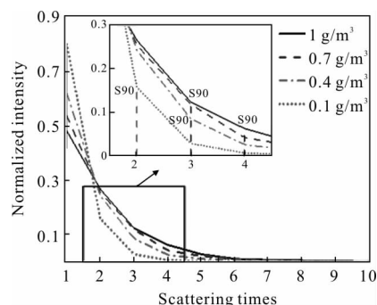
(a) 不同云雾质量浓度
