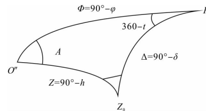
图 2 球面三角形
