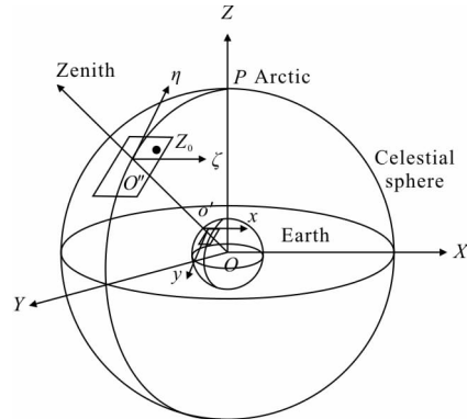
图 1 坐标系
