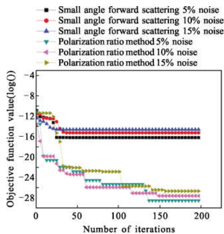
图 6 不同迭代次数下两种目标函数的函数值变化规律
