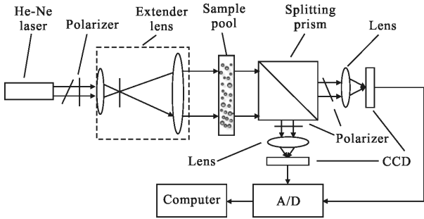
图 2 小角前向散射偏振比法系统原理图
