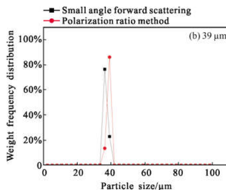
图 10 两种目标函数下 GBW(E) 120043(30 μm)和 GBW(E) 120028(39 μm)反演分布曲线
