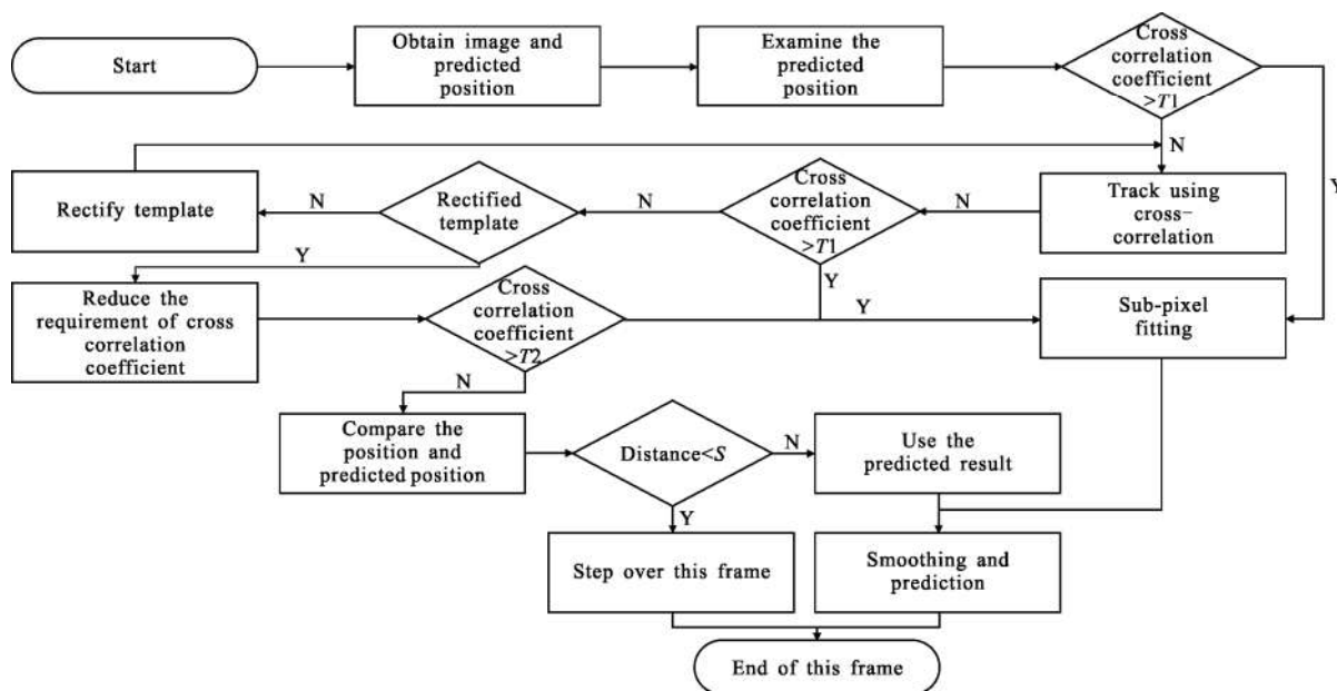
图5 算法流程
