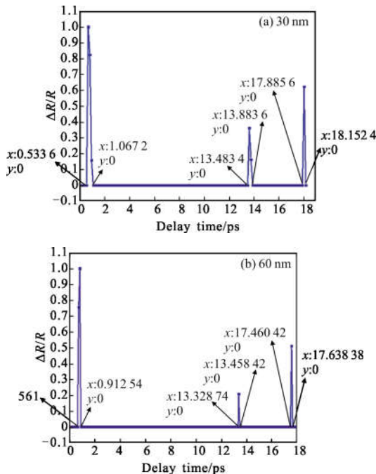
图 4 铜膜经三束飞秒激光辐照的实验结果
