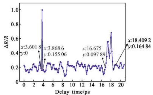
图 5 三束飞秒激光辐照 30\ \text{nm} 铜膜的实验结果
