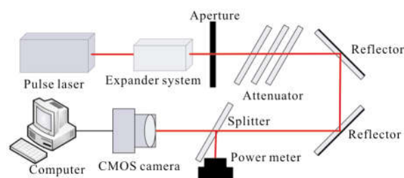
图 1 脉冲激光辐照 CMOS 相机实验布局示意图
