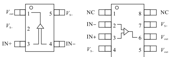
图 2 THS4303 器件封装形式
