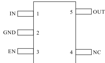
图 3 TPS760 器件封装形式
