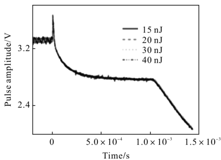
(a) 敏感位置 2 (a) Sensitive area 2#
