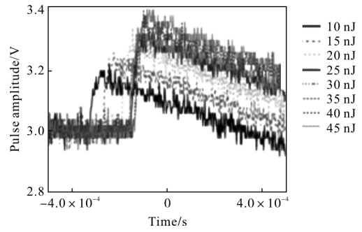
(b) 敏感位置 3 (b) Sensitive area 3#
