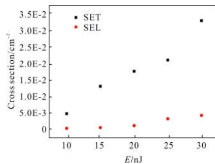
图 8 SEL 和瞬态 (SET) 截面随激光能量变化曲线
