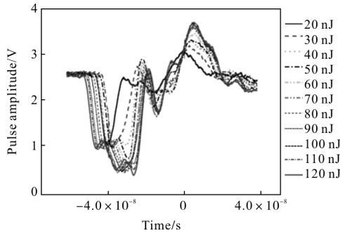
图 6 SET 波形随能量 E 的变化曲线(敏感位置 1)
