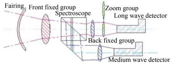
图 3 光学结构示意图
