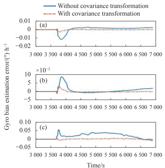
图 9 仿真实验中陀螺零偏相对估计误差
