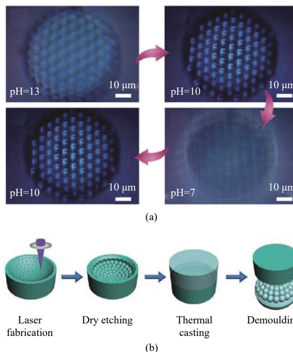
图 6 (a) 可变焦的仿生复眼 [6] ; (b) 蓝宝石凹面复眼模板及 K9 玻璃复眼制作原理图 [7]
