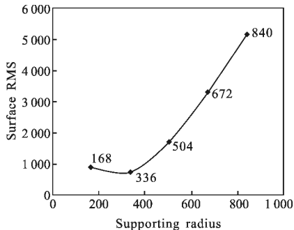
图 4 主镜镜面 RMS 随支撑半径变化曲线
