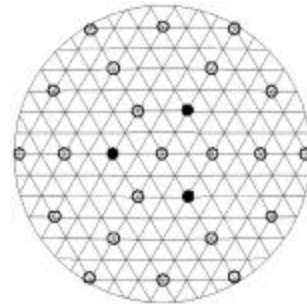
图 5 主镜支撑点及力驱动器布局
