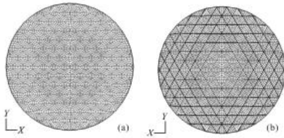
图 3 主镜有限元模型
