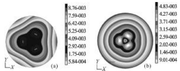
图 7 主镜在工况 2 作用下镜面变形云图
