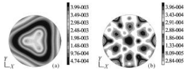
图 6 主镜在工况 1 作用下镜面变形云图
