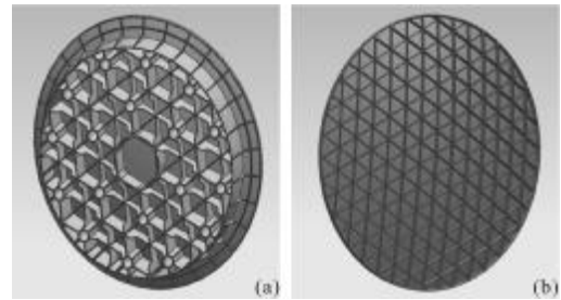
图 1 主镜结构形式
