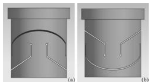
图 2 柔性支撑结构
