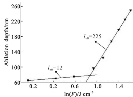
图 2 单脉冲 10 ps 激光烧蚀铝膜效率与能量密度的关系 [11]
