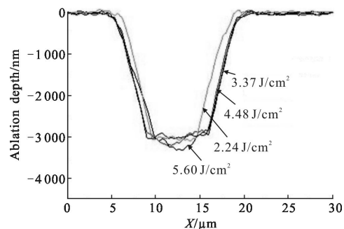
图 7 CGL 下,不同能量密度的激光重复加工多次烧蚀沟槽截面图
