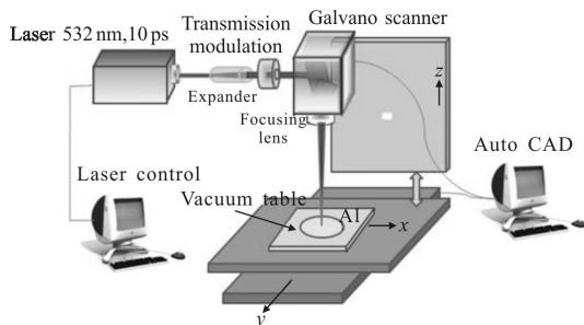
图 1 皮秒激光加工设备光学系统原理图
