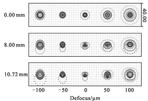
图3 可见光点列图
