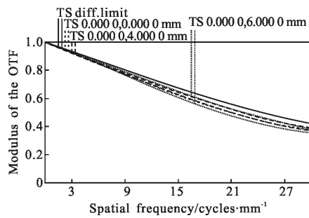
图 5 红外 MTF 曲线
