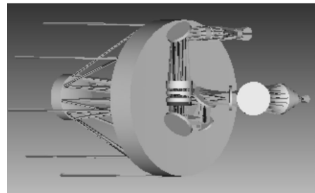
图1 光学系统布局
