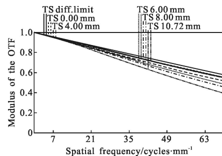
图2 可见光 MTF 曲线
