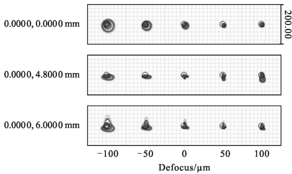
图 6 红外光点列图
