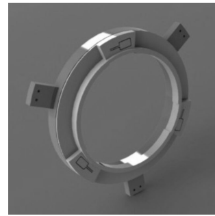
图 9 柔性支撑
