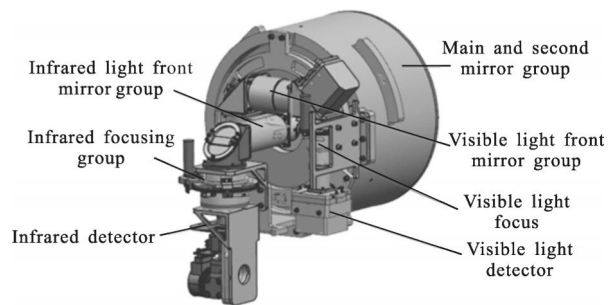
图 8 光机载荷三维图
