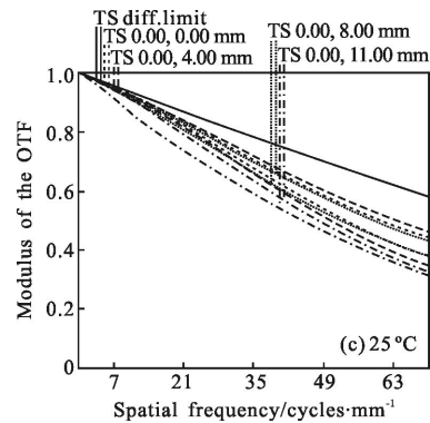
图 10 传函曲线
