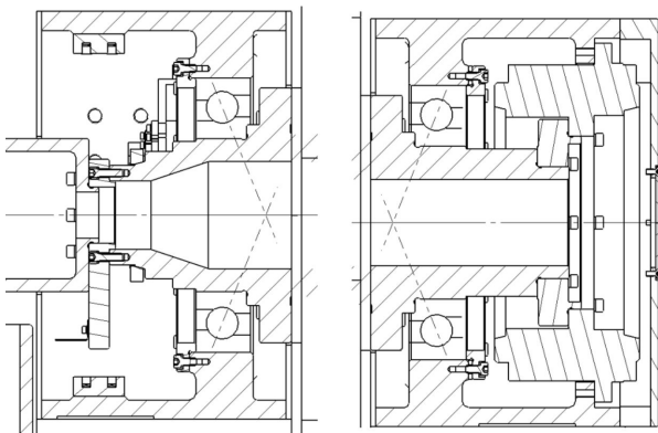
图 7 俯仰轴系结构设计图
