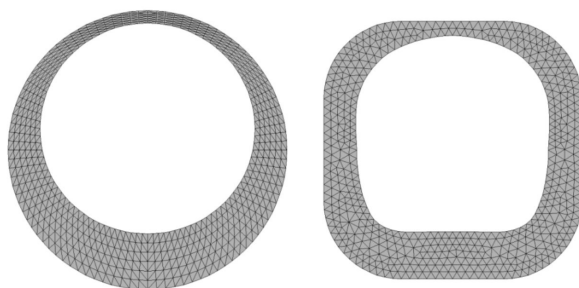
(a) 圆管 (a) Circular pipe (b) 方管 (b) Square pipe
