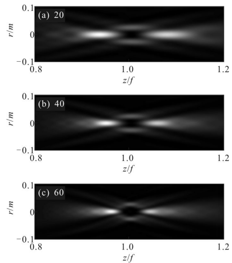
图 6 零阶贝塞尔高斯光束经菲涅尔波带片衍射后, 在焦点附近的光强分布
