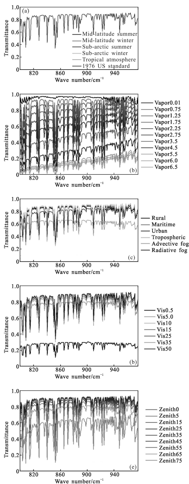
图1 不同变量对大气透过率光谱曲线的影响
