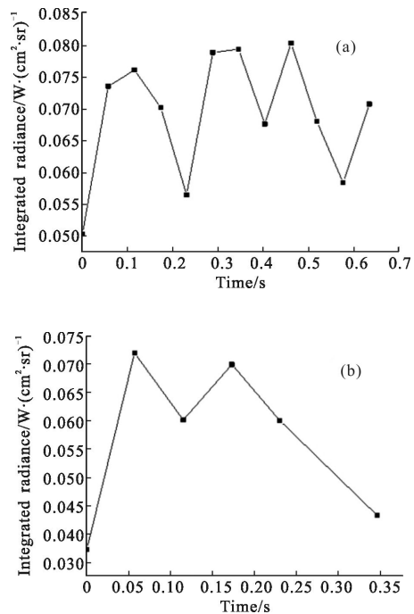
图 4 推进剂在波段范围内 ( 2000\sim 3333\text{ cm}^{-1} ) 的辐射亮度积分图
