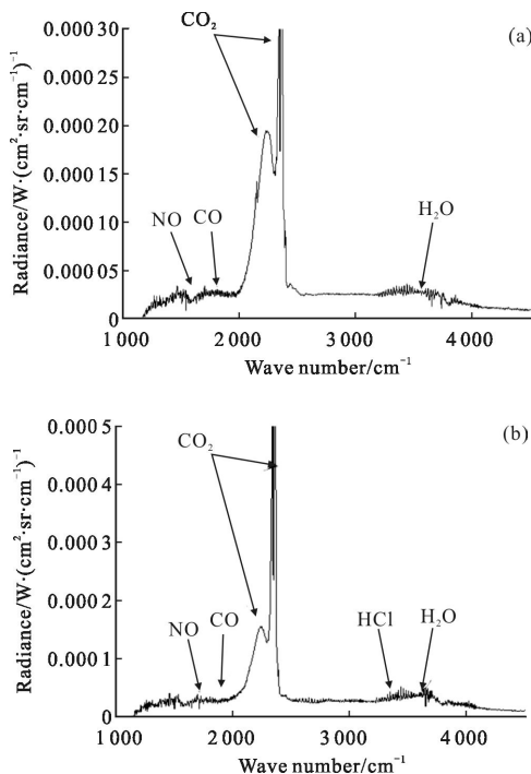
图 3 含 Al 推进剂和 NEPE 推进剂的红外辐射亮度图
