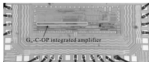
图 7 芯片照片
