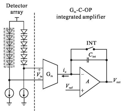
图 1 前端电路结构
