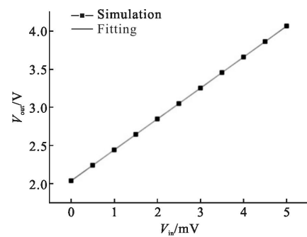
(b) 仿真与拟合曲线
