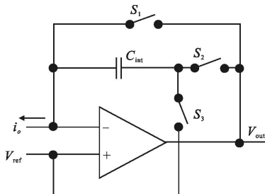
图 4 CTIA 结构图
