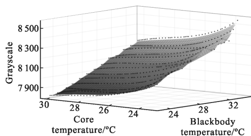
图 7 最小二乘法三阶拟合效果
