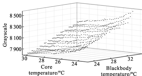
图 6 灰度随机芯温度和环境温度的变化曲线
