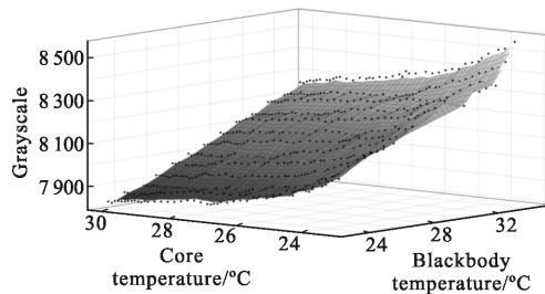
图 10 支持向量机拟合效果
