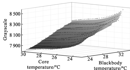
图 8 最小二乘法五阶拟合效果
