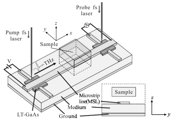
图 1 片上 THz 系统示意图
