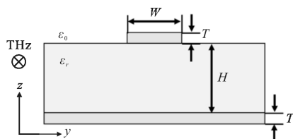
(a) 微带线横截面图及各参数定义
