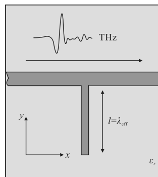
图 3 微带带阻滤波结构示意图
