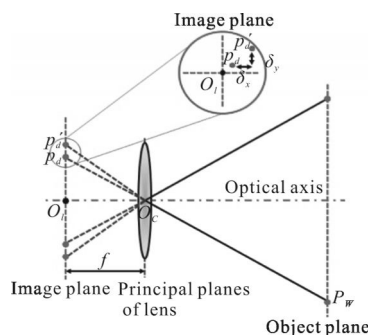
图 2 像机畸变原理图
