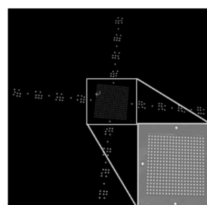
(a) 左相机拍摄靶标图像
