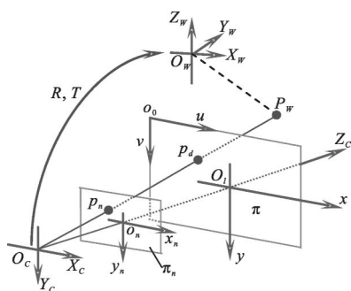
图 1 针孔摄像机模型示意图
