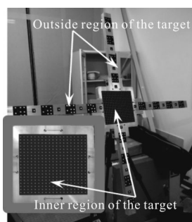
图 3 复合式靶标
