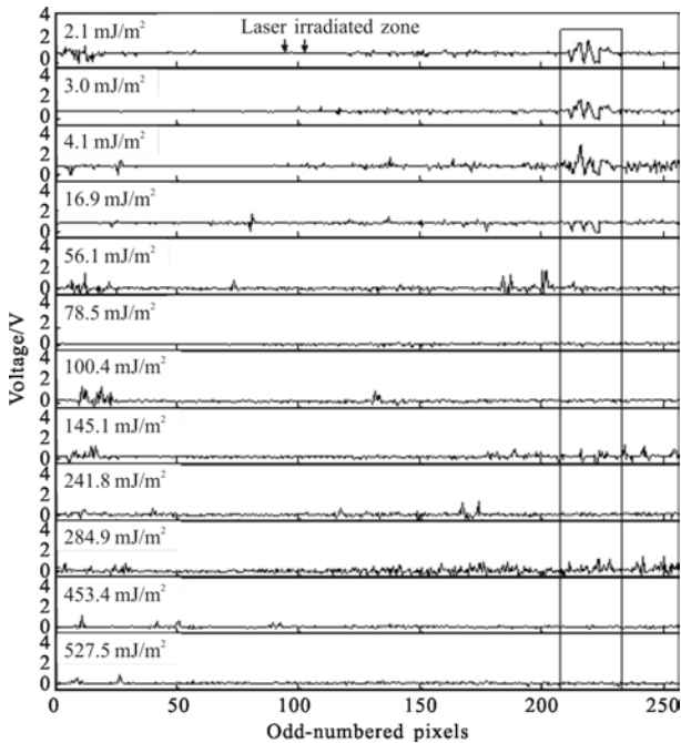
图 3 不同能量密度下探测器基底信号 V1 的响应曲线
