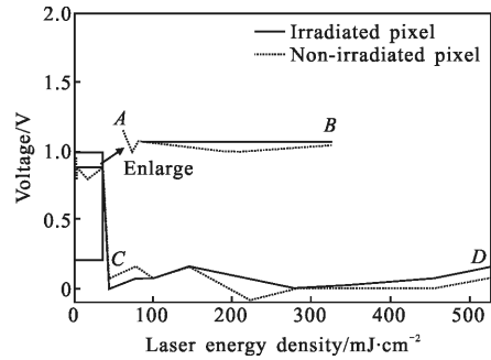
图 5 不同能量密度下被辐照、未被辐照像元的基底信号响应曲线
