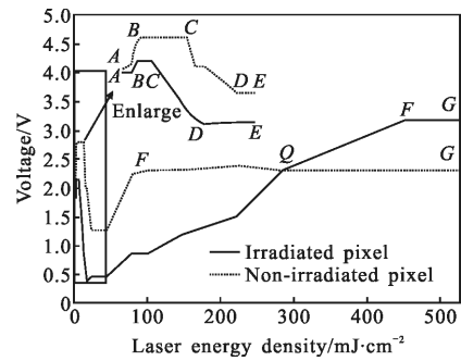
图 6 不同能量密度下被辐照、未被辐照像元的光响应信号曲线
