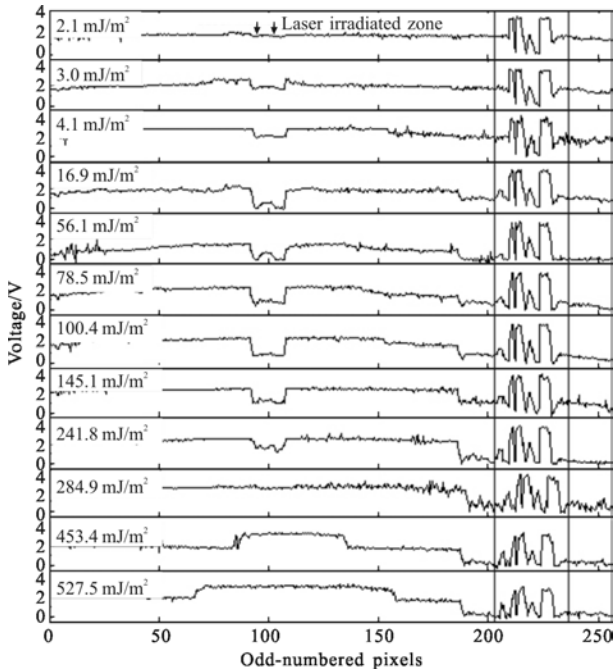
图 4 不同能量密度下探测器奇光响应信号 V2 的响应曲线
