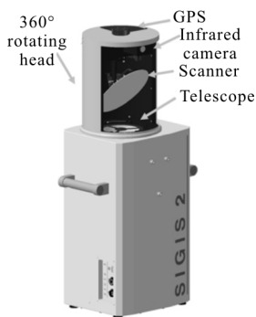
图 3 Bruker SIGIS2 红外光谱仪
