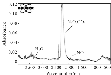
图 12 尾焰流场检测出的燃烧产物
