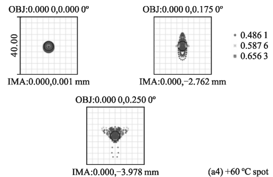
(a) -40^\circ\text{C} 、 +60^\circ\text{C} 时可见光系统的调制函数曲线和点列图
