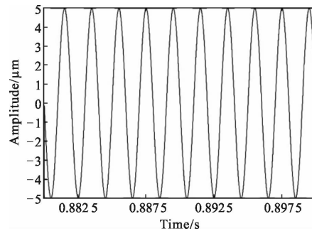
图 4 解调输出结果
