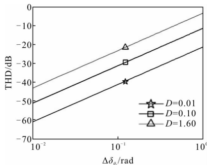
图 2 \text{THD}_{\max} 与相位延迟 \Delta\delta_{\theta} 的关系 Fig.2 Relations of \text{THD}_{\max} and \Delta\delta_{\theta}
