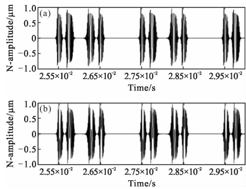
图 3 两路干涉信号
