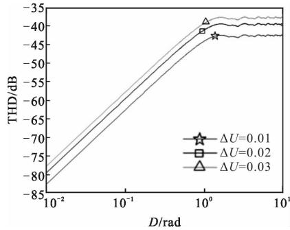
图 1 \text{THD}_{\max} 与输入信号幅值 D 的关系 Fig.1 Relations of \text{THD}_{\max} and D
