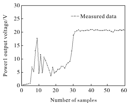
图 10 加算法时 Power1 的输出电压
