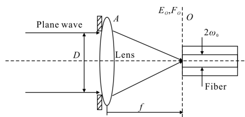
图 1 光纤耦合原理图
