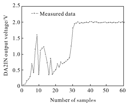
图 9 加算法时 DA2IN 电压
