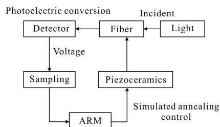
图 2 空间光-光纤耦合自动对准系统
