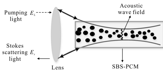
图 2 SBS 系统物理场景
