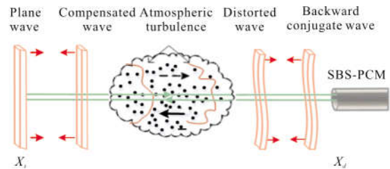
图 1 相位共轭镜修正波前畸变过程
