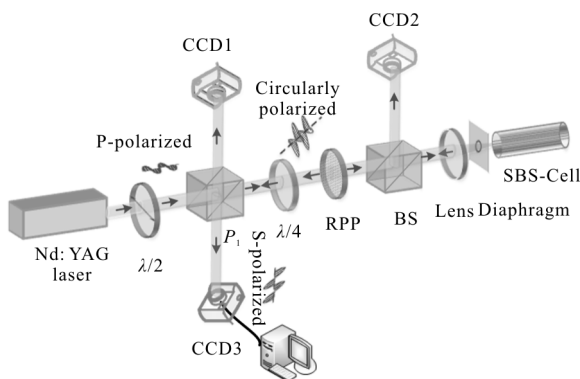
图 5 实验装置图 Fig.5 Experimental setup
