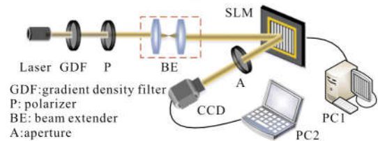
图 3 实验装置图
