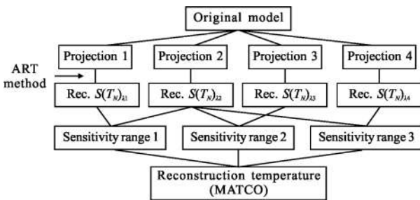
图 4 多条吸收谱线组合优化方法流程图
