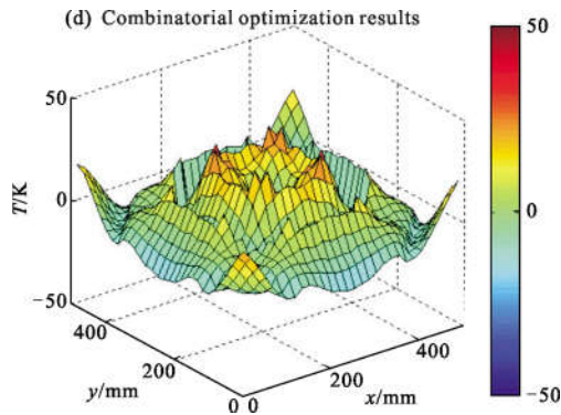
图 5 温度场重建结果与原始温度分布的比较
