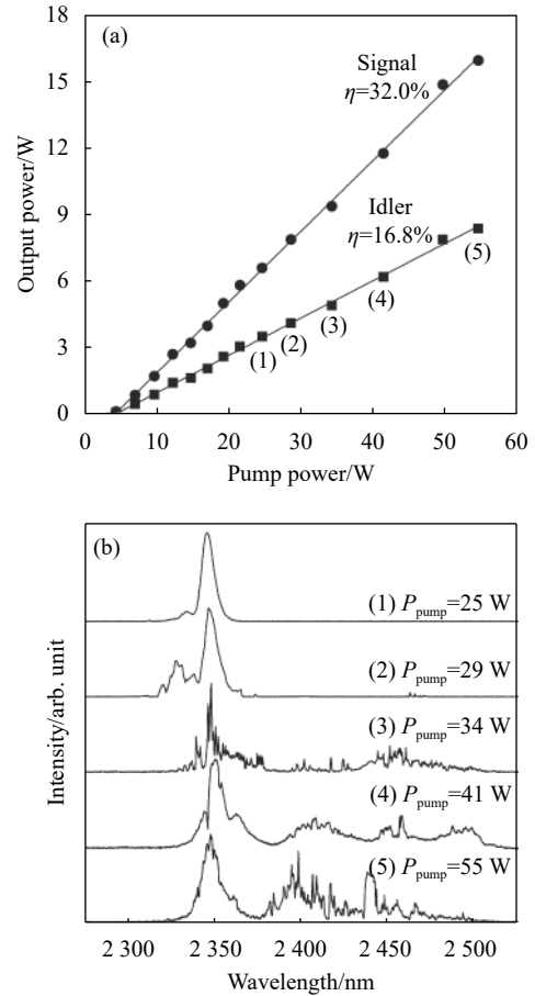
图 2 腔内无 LiNbO 3 时的 OPO 输出特性: (a) 信号光和闲频光功率随泵浦功率的变化; (b) 闲频光光谱随泵浦功率的变化
