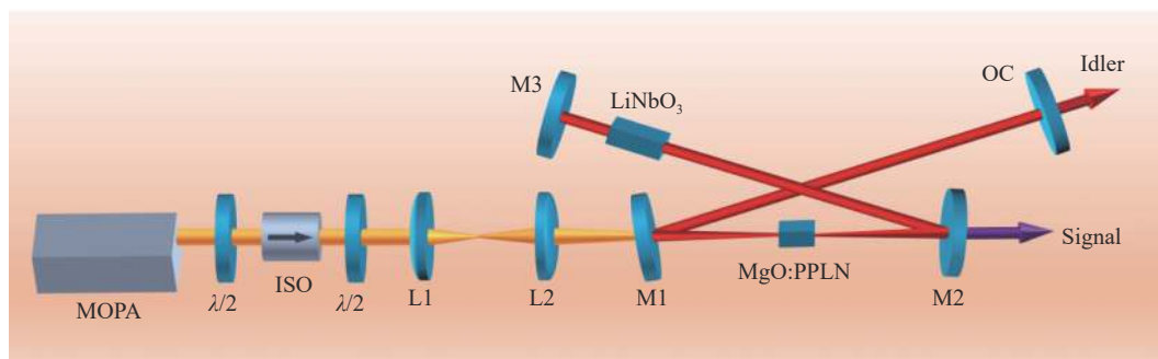
图 1 基于色散管理实现光谱净化和稳定性提升的飞秒 OPO 装置
