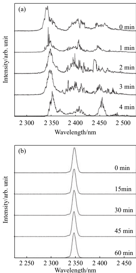
图 3 腔内不插入 (a) 和插入 (b) LiNbO 3 晶体时闲频光光谱随时间的变化
