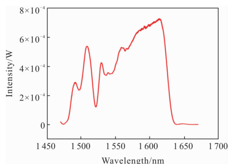
图 3 光源的光谱
