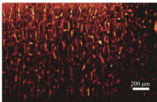
图 10 新鲜洋葱组织内部 500 μm 成像深度大范围激光回馈共聚焦层析图像
