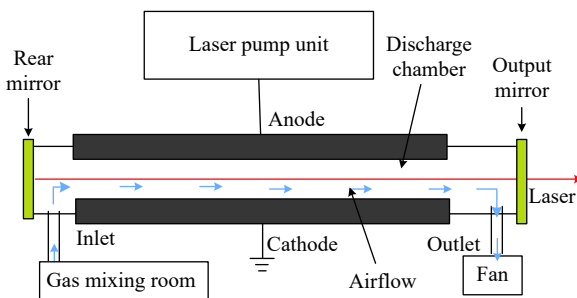
图 1 激光器系统截面示意图
