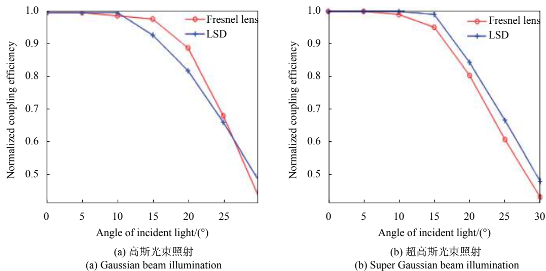
图 4 耦合效率随激光入射角的变化
