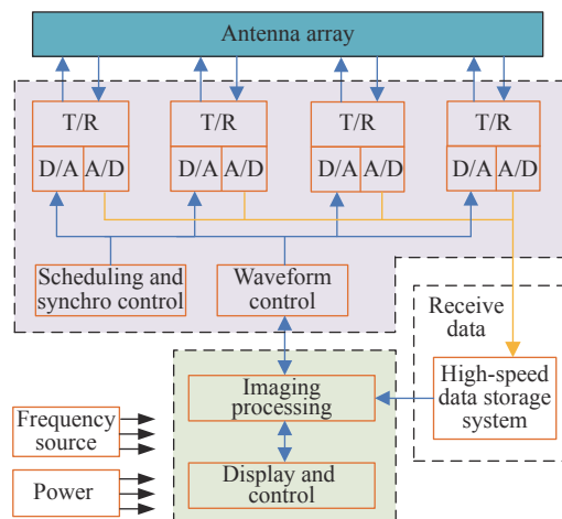
图 17 数字阵列微波关联成像系统通用结构图 [15]
