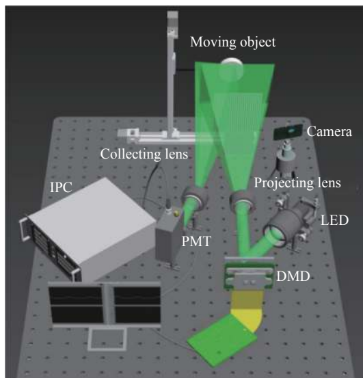
图 4 实验系统图
