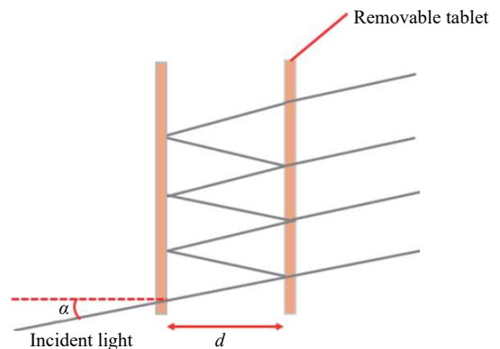
图 6 超窄线宽滤波器原理图
